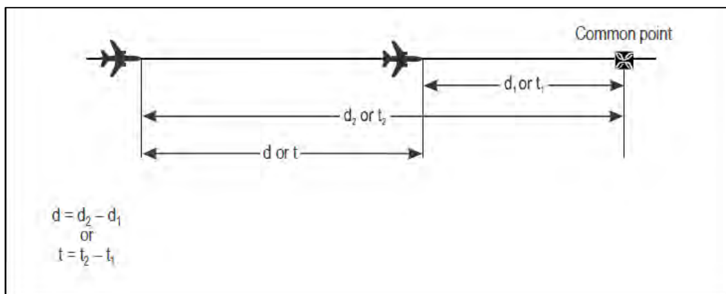
Figura 5-30. Cálculo de la distancia/tiempo longitudinal entre aeronaves — derrota idéntica, mismo sentido [véase 5.4.2.9.5 a)]
