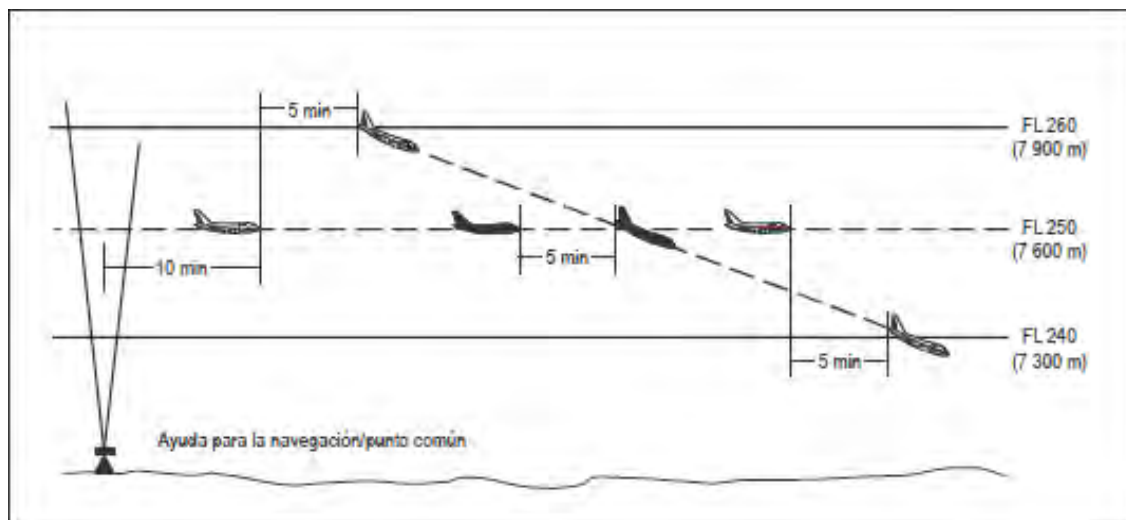
Figura 5-18B Separación de 5 minutos entre aeronaves que descienden y por la misma derrota [véase 5.4.2.2.1 c) 2)]
