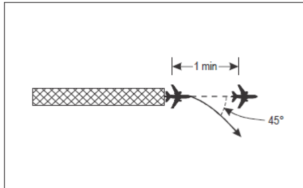
Figura 5-37 Un minuto de separación entre aeronaves que salen y siguen derrotas divergentes por lo menos en 45^\circ [véase 5.6.1]
