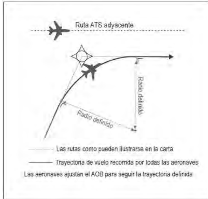
Transición de radio fijo (FTR)
