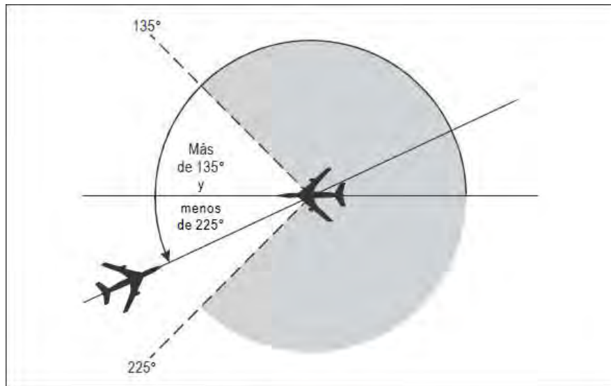
Figura 5-8 Aeronaves por derrotas opuestas [véase 5.4.2.1.5 b)]
