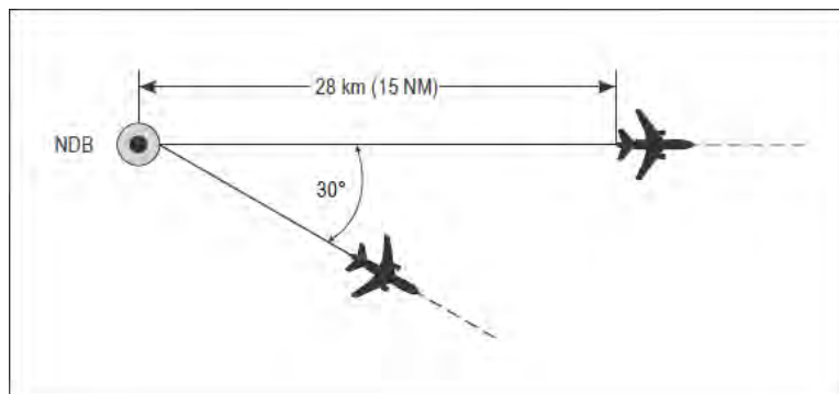
Figura 5-5 Separación utilizando el mismo NDB
