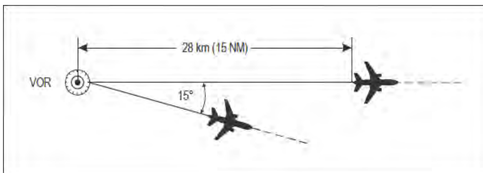
Figura 5-4.4 Separación utilizando el mismo VOR
