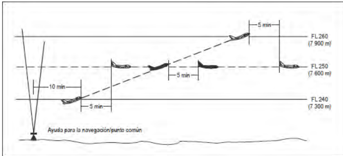
Figura 5-18A Separación de 5 minutos entre aeronaves que ascienden y por la misma derrota [véase 5.4.2.2.1 c) 2)]
