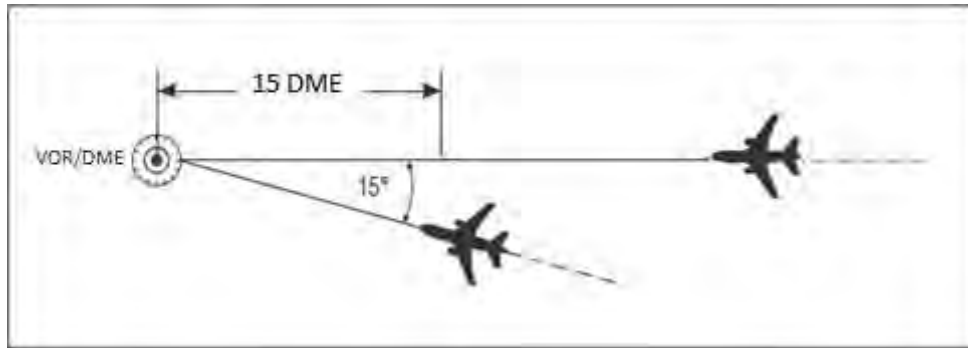
Figura 5-4.2 Separación utilizando el mismo VOR/DME
