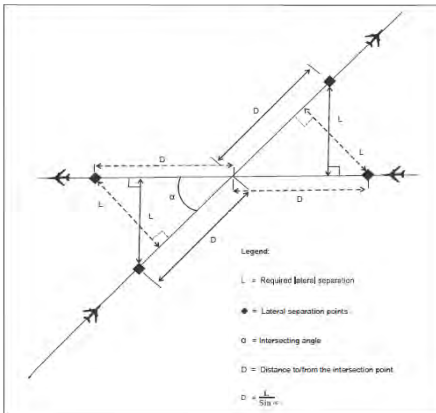
Figura 5-6 Puntos de separación lateral (véase 5.4.1.2.1.7)
