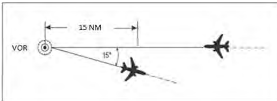
Figura 5-4.6 Separación utilizando el mismo VOR
