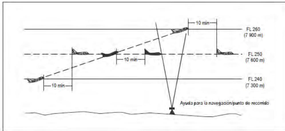
Figura 5-17A Separación de 10 minutos entre aeronaves que ascienden y por la misma derrota [véase 5.4.2.2.2.1 b)]
