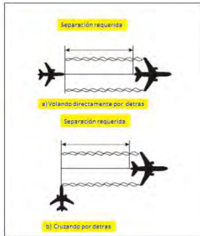
Figura 8-1 Vuelo directamente por detrás o cruce por detrás (véanse 8.7.3.4 y 8.7.3.5)
