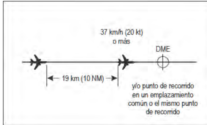
Figura 5-23. Separación de 10NM basada en DME o GNSS
