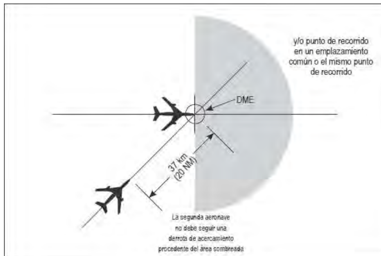
Figura 5-24A. Separación de 20NM basada en DME o GNSS
