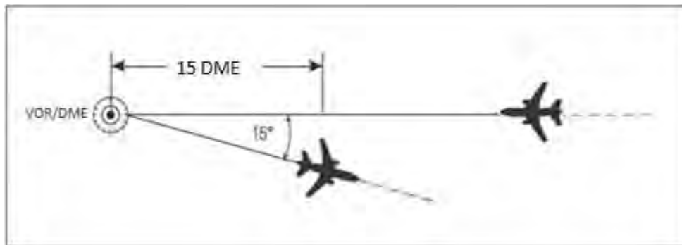
Figura 5-4.3 Separación utilizando el mismo VOR/DME
