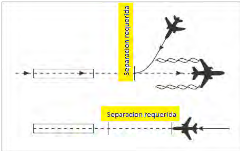
Figura 5-46 Separación por estela turbulenta para aterrizaje en sentidos opuestos [véanse 5.8.5.1 b) y 5.8.5.2 b)]
