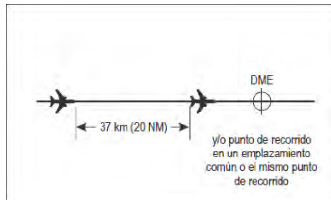
Figura 5-22. Separación de 20NM basada en DME o GNSS
