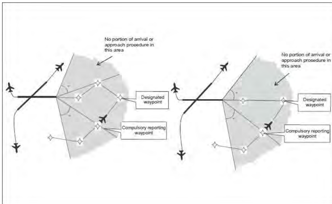
Figura 5-41. Área de protección de llegada
