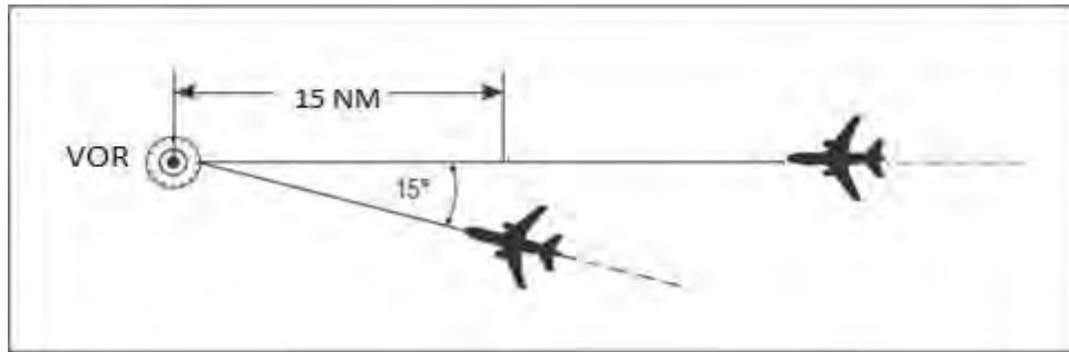
Figura 5-4.5 Separación utilizando el mismo VOR
