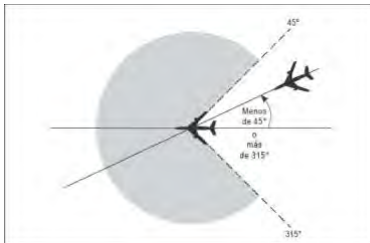
Figura 5-7 Aeronaves por la misma derrota [véase 5.4.2.1.5 a)]
